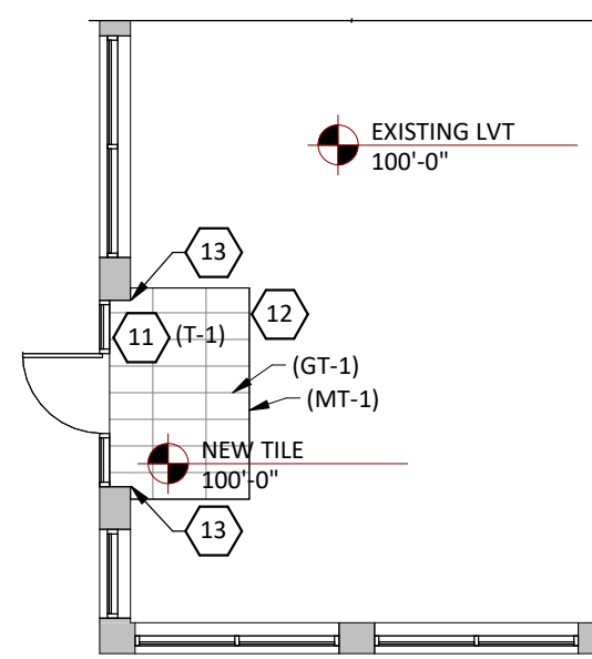
3B VESTIBULE PLAN A301 SCALE: 1/8" = 1'-0"
