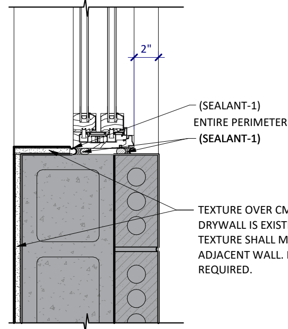
3B A311 WINDOW JAMB DETAIL SCALE: 1 1/2" = 1'-0"
